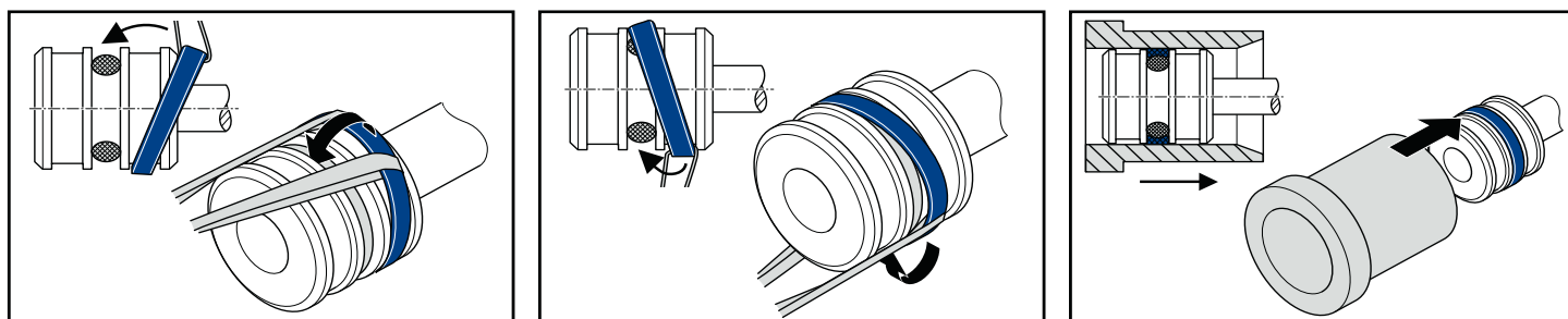
2. Einbau mit Montageband und Kalibrierhülse | Installazione con nastro di montaggio e manicotto di calibratura | Montering med monteringsband och kalibreringshylsa | Montage met tape en kalibreerbus
