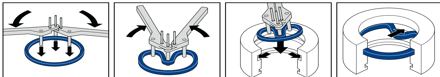
1A. Einbau mit Montagezange | Installazione con pinza di montaggio | Montering med monteringsstång | Montage met een tang
