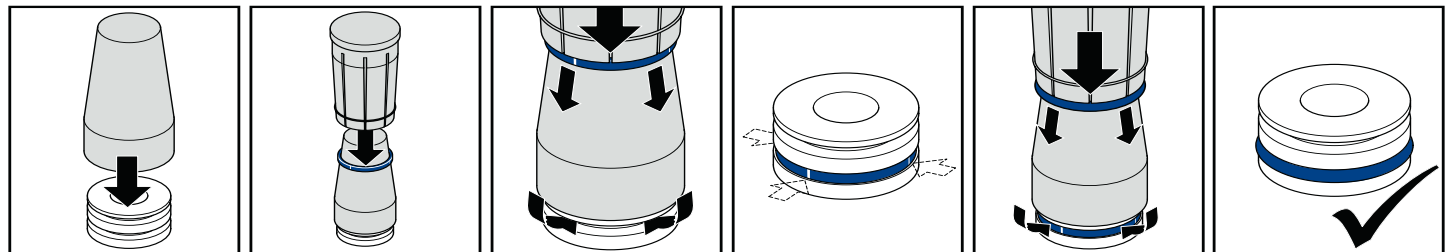
1. Einbau mit Spreizdüse und Montagekegel | Costruito con mandrino di espansione e cono di montaggio | Montering med slitsad monteringshylsa och montagekona | Montage met spreidstuk en Montagekegel
