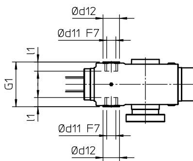
Attacco posteriore BOCCOLE Config.3
