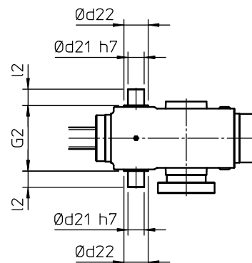
Attacco posteriore PERNI Config.4
