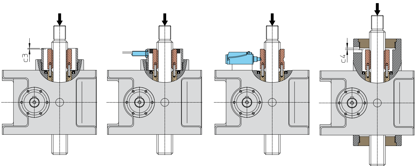
Controllo usura filetto su martinetti Serie MA Mod.A
