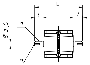
Vers.2: Doppio albero entrata
