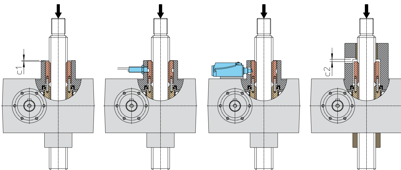
Controllo usura filetto su martinetti Serie SJ Mod.A
