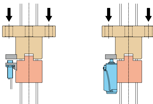
Controllo usura filetto su martinetti Serie SJ Mod.B
