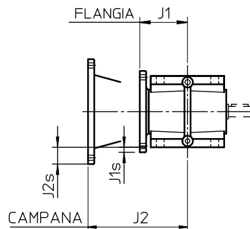
Vers.5: Vers.1 con campana e giunto IEC
